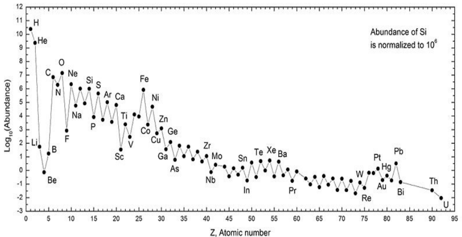
太阳系前 92 种化学元素的丰度
